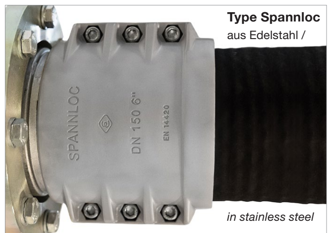
Type DFC mit eingekammerter Profildichtung with captive seal
